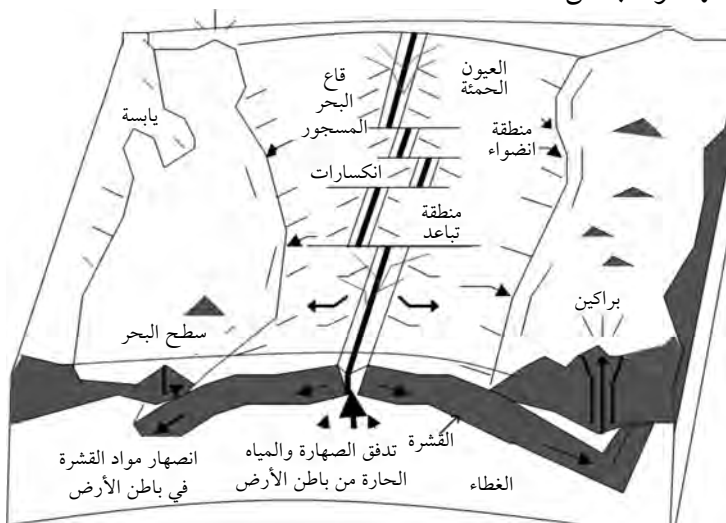
الشكل ١٣: مظهر لحركية القمع المكونة لسطح الأرض.
