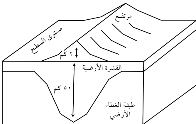
الشكل ١١: يبين القشرة الأرضية أكثر سمكاً تحت المرتفعات. وارتفاع سمك القشرة تحت الجبل يدل على كونه موثداً في الأرض.
