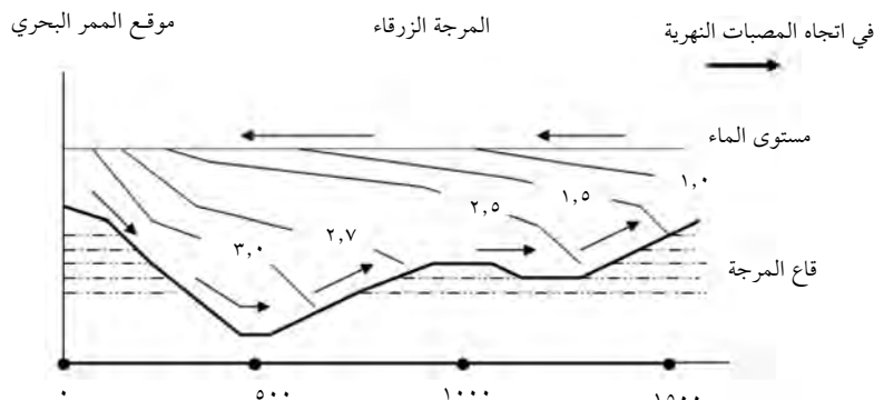
الشكل ١٦: يبين المستويات الفاصلة بين الكتل المائيّة مختلفة الملوحة من الممرّ البحري إلى المصبّ النهرية. الأرقام تبيّن النسبة المئوية للملوحة. السهام (←) تبيّن اتجاه التيارات المائيّة في المرجة.
